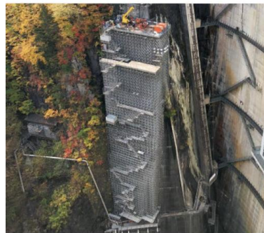
YT ロックシステム システム構台
